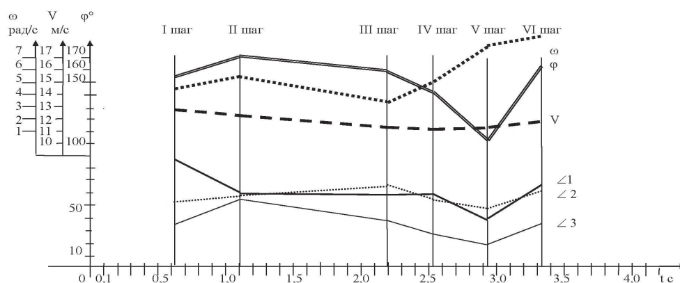
Рисунок 1 – Изменение угловых параметров и скорости в скользящем шаге при беге по повороту на дистанции 500 метров
